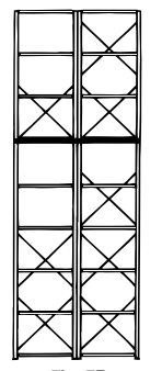
Fig. 7B Side Brace
