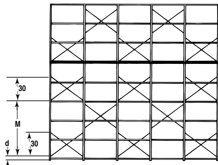
Fig. 5 Back Brace
