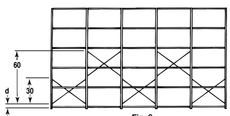
Fig. 6 Back Brace
